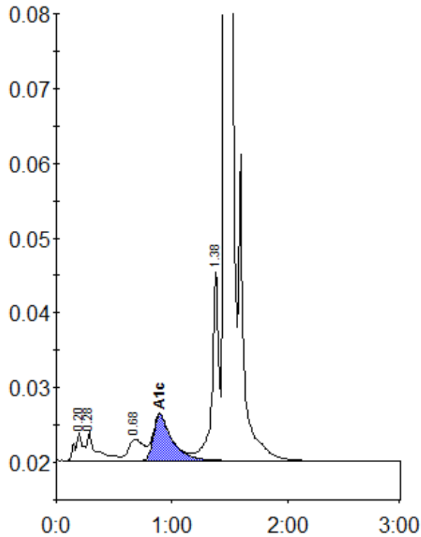
Peak table - ID: 10364973
